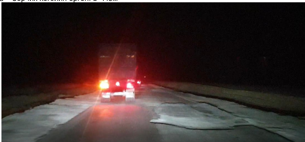
Зураг №3.Гашуун сухайт чиглэлийн автозамын хөвөө, далан, усны шуудуу зэргийн эвдэрсэн байдал (2022/09/15)
